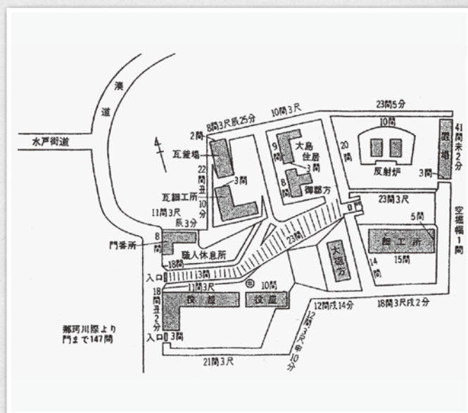
反射炉施設配置図(安政元年「湊村反射炉場所図」より作成(『金風』1968年10月1日号より))
